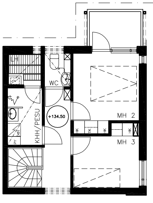
2. KERROS
